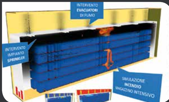
Simulazione di incendio in un deposito ad alto impilamento
